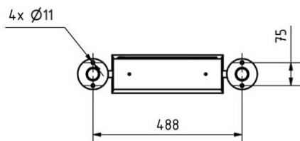
Montagebohrungen
