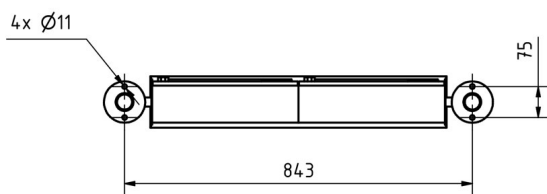
Montagebohrungen
