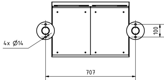
Montagebohrungen
