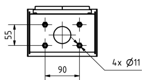
Montagebohrungen
