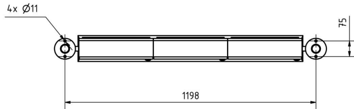
Montagebohrungen
