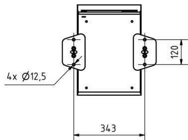
Montagebohrungen
