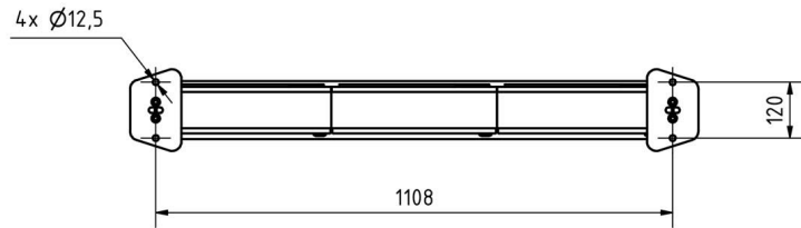
Montagebohrungen
