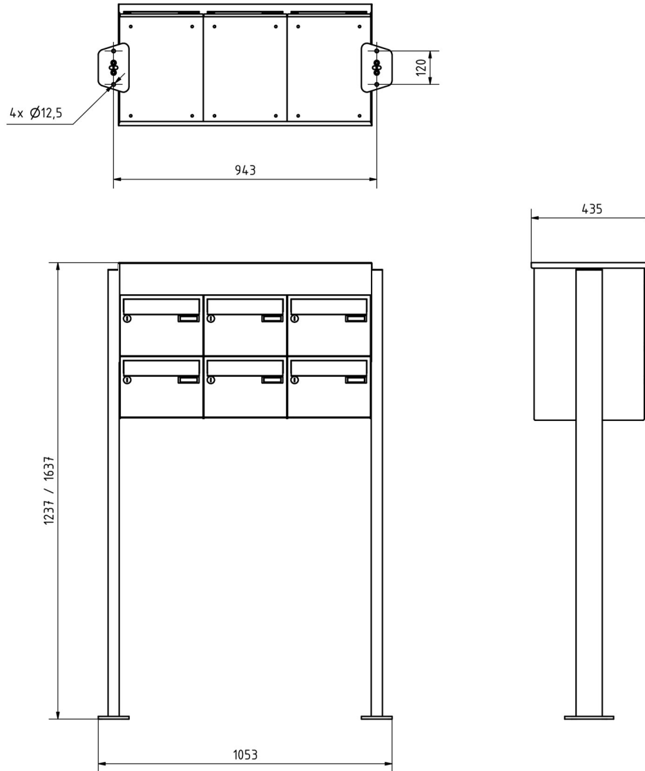
Montagebohrungen
