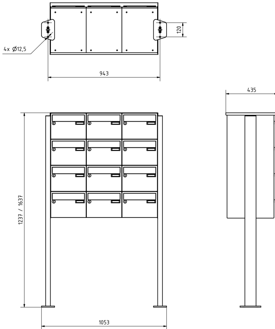
Montagebohrungen
