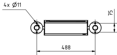
Montagebohrungen
