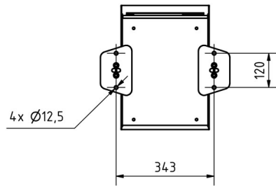
Montagebohrungen
