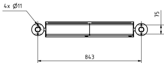
Montagebohrungen
