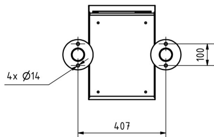
Montagebohrungen
