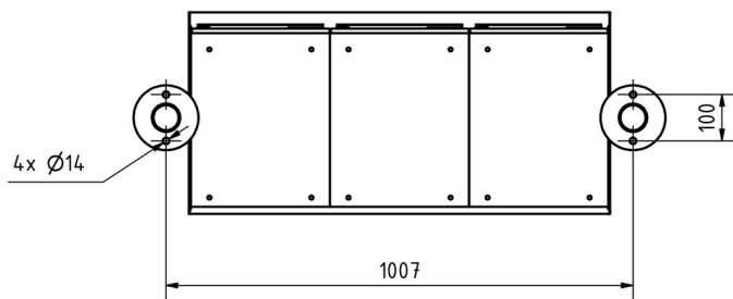
Montagebohrungen
