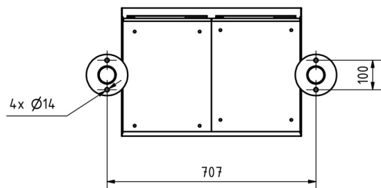
Montagebohrungen
