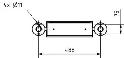
Montagebohrungen
