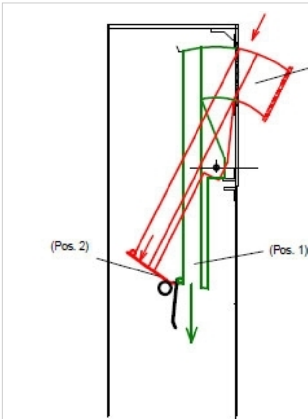
Prinzip der Schleusentechnik ( gebrauchsmustergeschützt )
