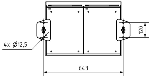
Montagebohrungen
