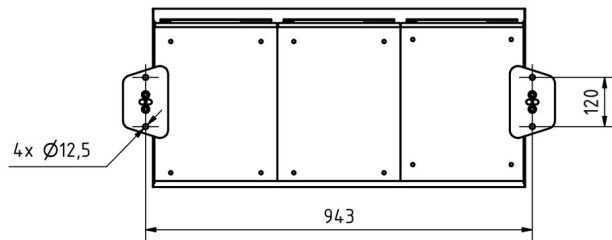
Montagebohrungen
