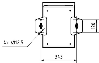
Montagebohrungen
