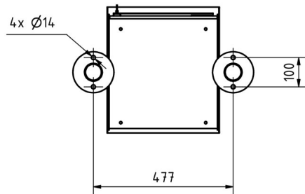
Montagebohrungen
