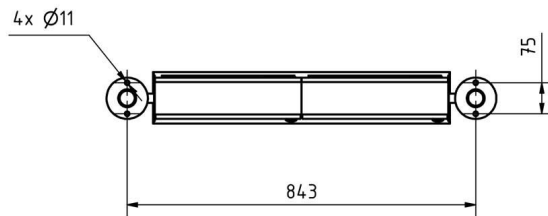
Montagebohrungen
