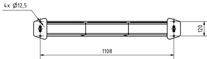
Montagebohrungen
