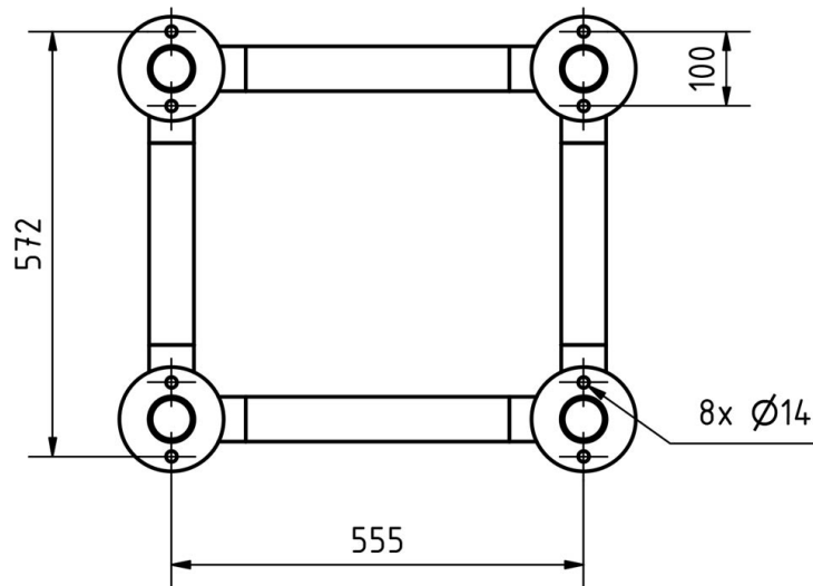
Montagebohrung
