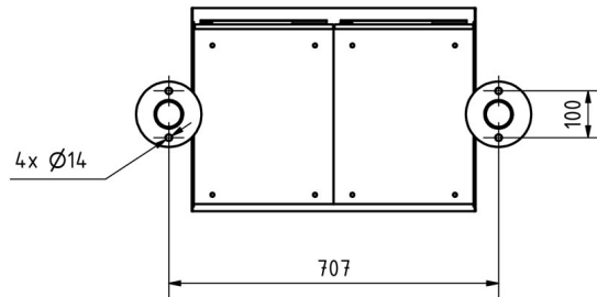
Montagebohrungen
