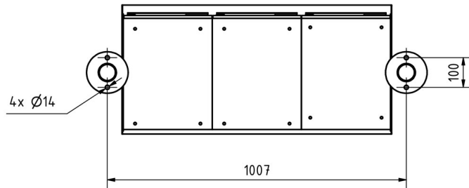
Montagebohrungen
