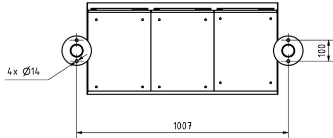
Montagebohrungen
