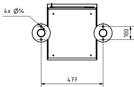
Montagebohrungen
