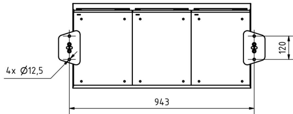
Montagebohrungen
