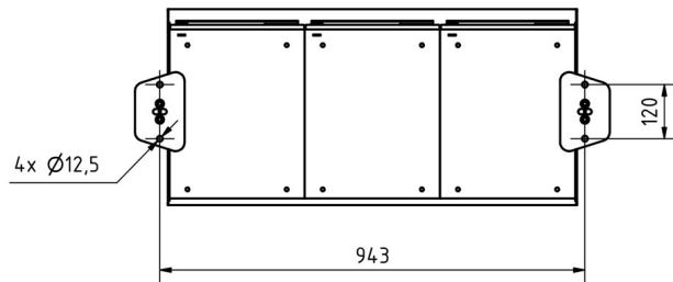
Montagebohrungen
