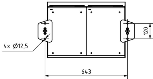
Montagebohrungen
