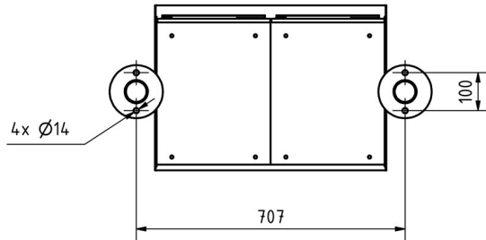
Montagebohrungen
